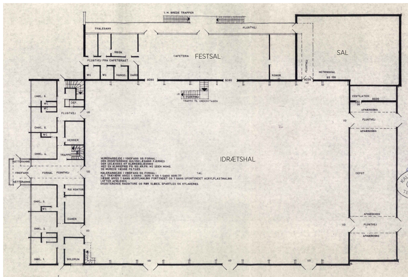
Grundplan af den eksisterende Røsnæshal
